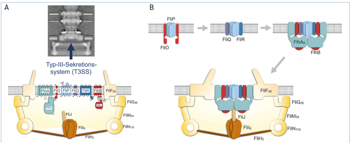
▲ Abb. 2: Koordinierter Aufbau des flagellumspezifischen Typ-III-Sekretionssystems (T3SS). A, elektronenmikroskopische Aufnahme des Basalkörpers von Flagellen (oben; mit freundlicher Genehmigung von David DeRosier, modifiziert nach [13]) und schematische Darstellung des T3SS von Flagellen (unten). Das T3SS besteht aus sechs Membranproteinen, einem cytoplasmatischen ATPase-Komplex und einem cytoplasmatischen Ring, welcher eine duale Funktion als Rotor des Flagellums sowie in der Bindung von T3SS-Substraten hat. Blauer Pfeil: Position des T3SS in der inneren Membran. B, Modell, wie das flagellumspezifische Chaperon FliO den Aufbau des zentralen Porenkomplexes des T3SS koordiniert. Das Chaperon FliO interagiert mit dem Porenprotein FliP und ermöglicht die Bildung eines stabilen Porenkomplexes. FliO wird durch andere Membranbestandteile des T3SS (FliQ und FliR) ersetzt, nachdem ein stabiler FliP-Komplex gebildet wurde. Die Bildung eines Porenkomplexes aus FliP-FliQ-FliR ist die Grundlage für den weiteren Aufbau eines funktionalen T3SS (© M. Erhardt).
